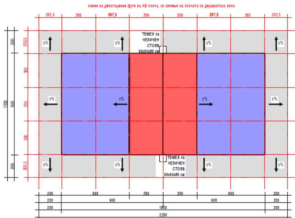
figurë 10 Pamje skematike e sheshit të lojërave të basketbollit
