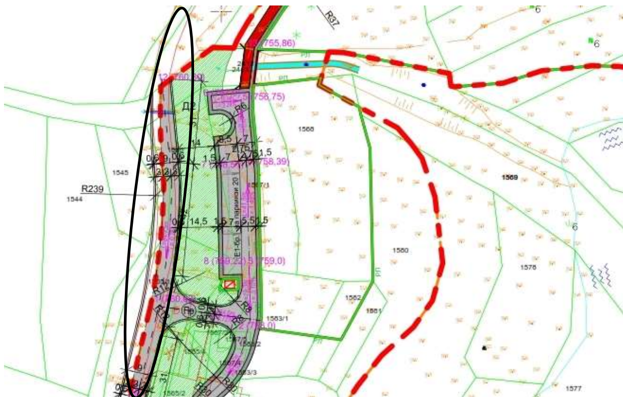
figurë 4 Pamje skematike e rrugës Rajonal (e shënuar me të zezë), rruga hyrëse dhe hapësira e parkimit (Zona e shënuar me të verdhë është zona ekzistuese e parkimit, ku është planifikuar rregullimi i rrugës hyrëse dhe parkimit.)
