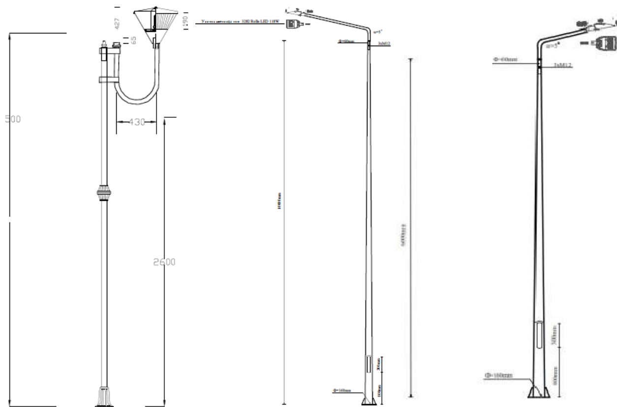
figurë 9 Paraqitje i dy modeleve të candelabras
