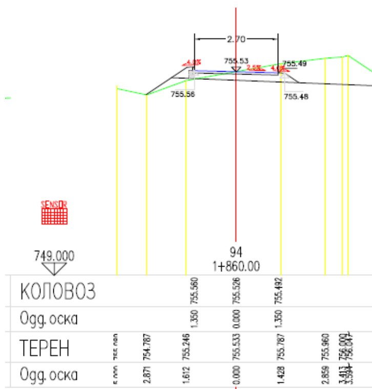
figurë 3 Profil i tërthortë i shtegu për biçikletës
