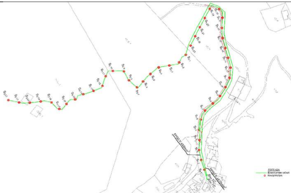
Figura 12 Pamje skematike e pozicioneve ku do të montohet Dritat nga shtëpia e gjuetarëve deti te Kulla e Mbretit
