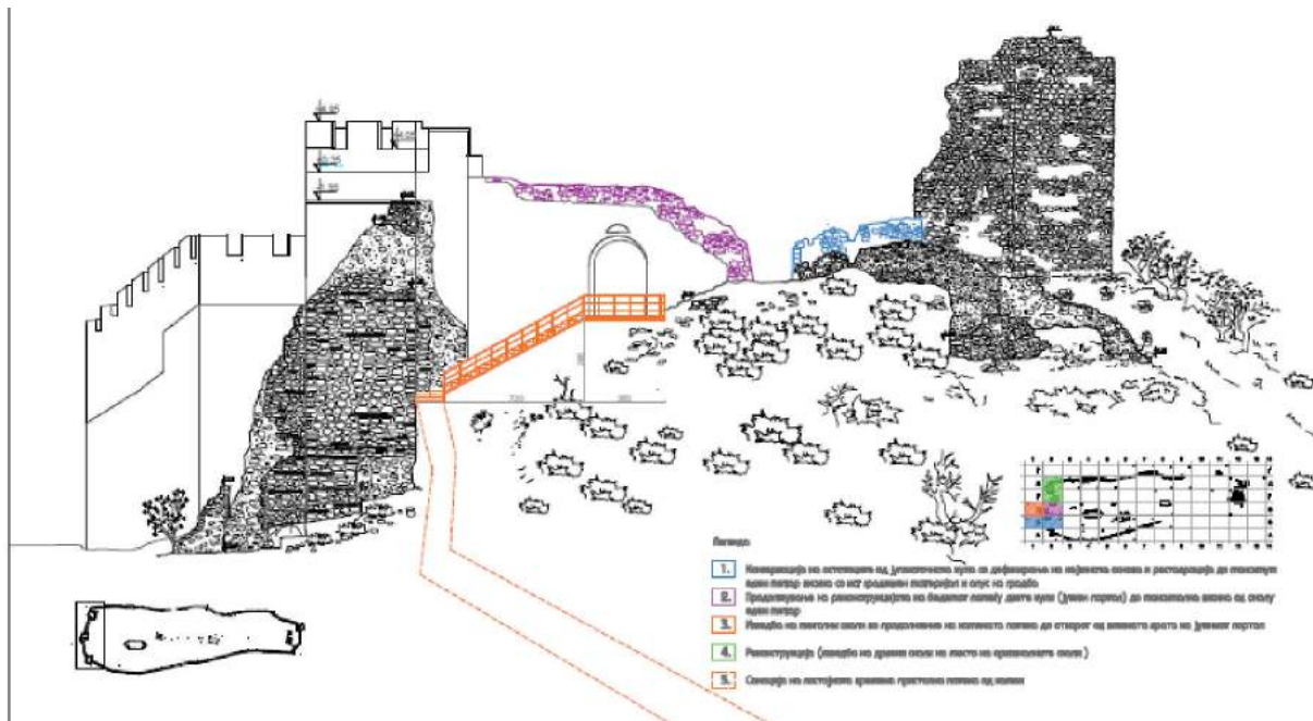
Foto 8 Paraqitja e pjesës jugore dhe kullës jug-lindore me ndërhyrje
