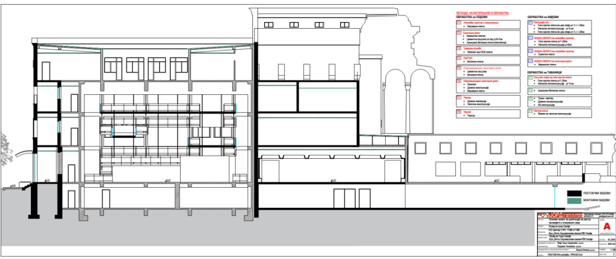
Слика 8 Пресек на сегашната состојба Б-Б
